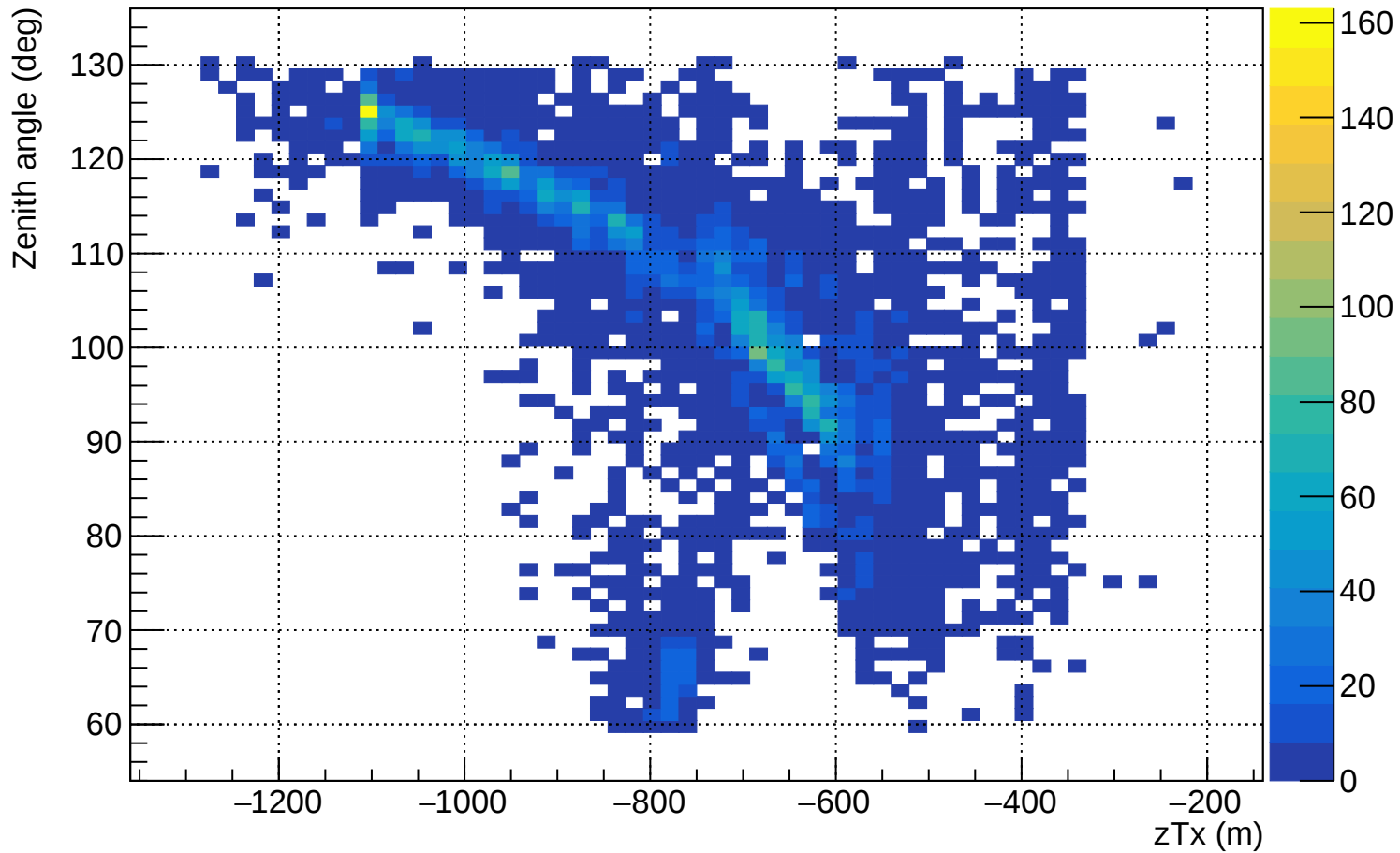
A1 Z4Vtx zenith angle
