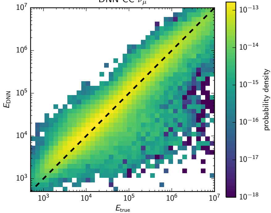
DNN CC \nu_\mu
